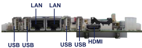
3I280CM-HRH2 Rear I/O
